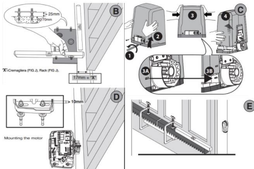
Sơ đồ lắp đặt thiết bị motor cổng trượt Deimos A400
